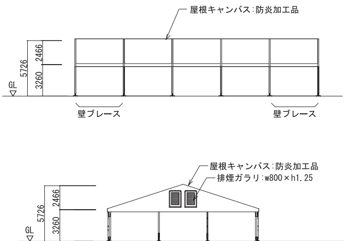
立面図
