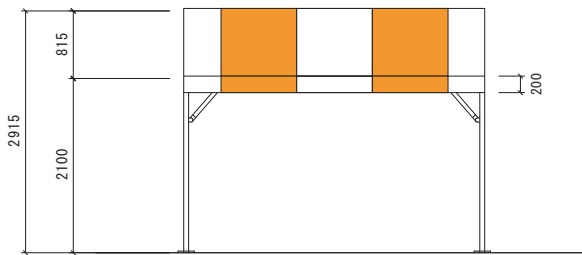
断面図
